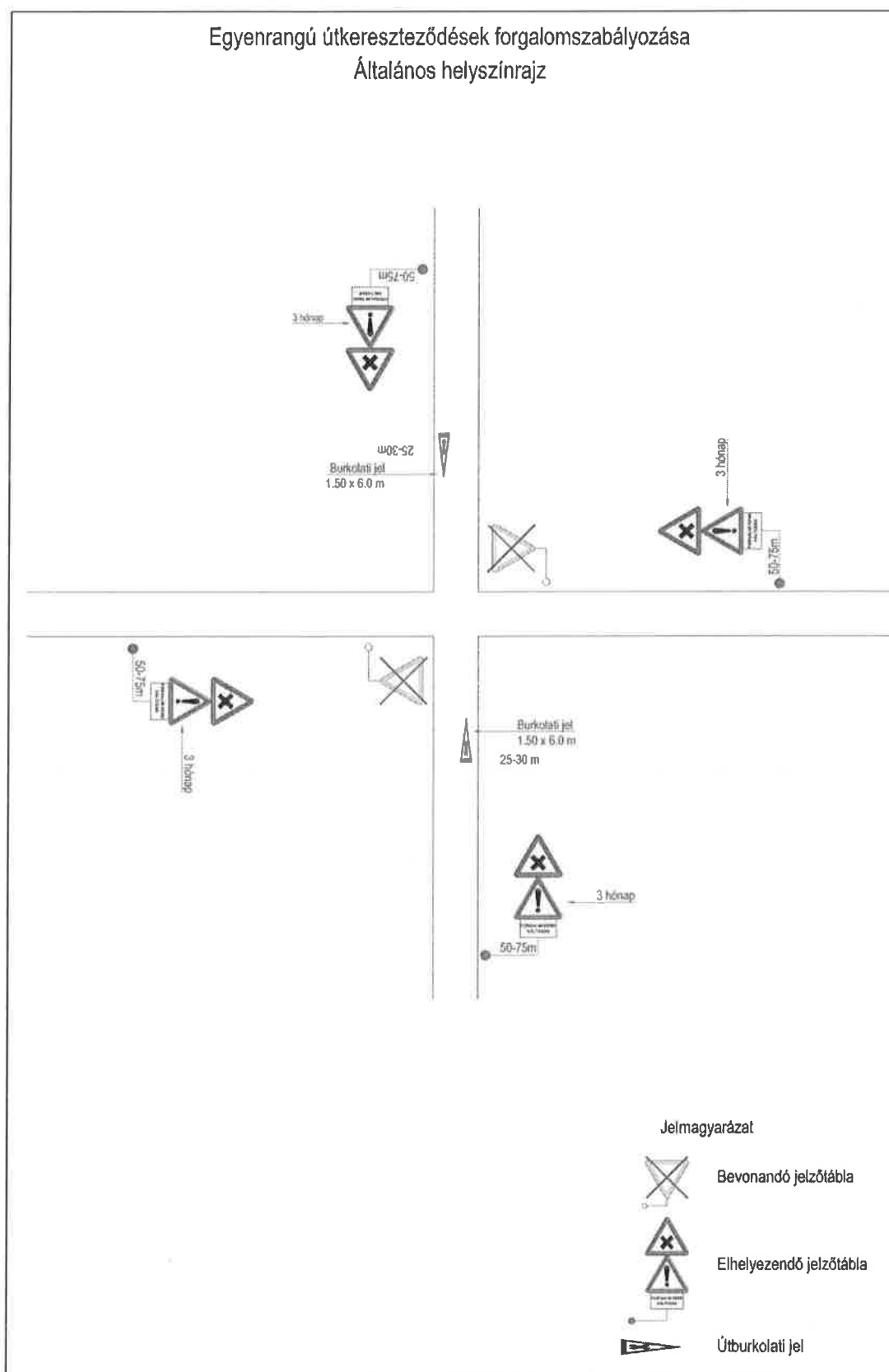
2. ábra: Általános helyszínrajz: Egyenrangú útkereszteződések elsőbbség szabályozása
