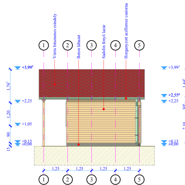
É-3 Keleti homlokzat 1:100
