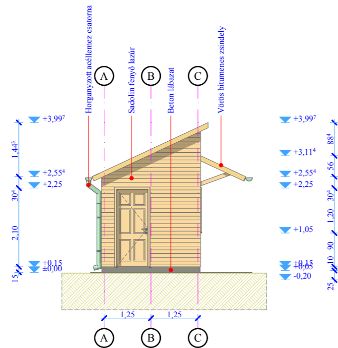
É-3 Északi homlokzat 1:100
