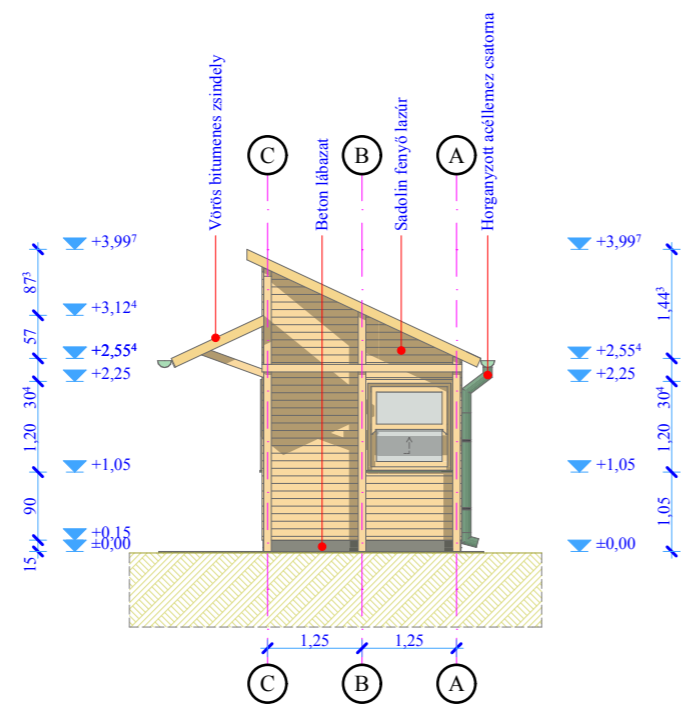
É-3 Déli homlokzat 1:100
