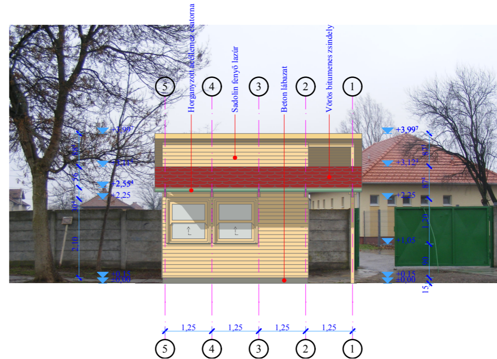
É-3 Nyugati homlokzat 1:100
